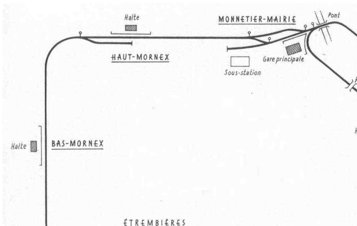
Fig. 02 - Évitements, aiguillages, gares, haltes et correspondances avec les autres chemins de fer (dessin de Pierre Duvernay selon les informations de G. Lepère).
