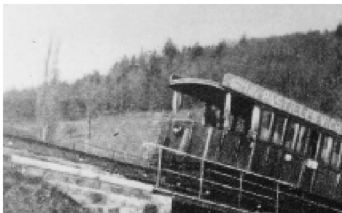
Fig. 19 - Une automotrice (2 e époque) franchit le pont n° 15 en amont de la halte de Haut-Mornex ; au fond le sommet du mont Gosse.
